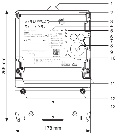
Vorderansicht
